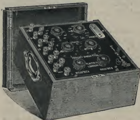
Fig. 775.—Barretter Apparatus.
