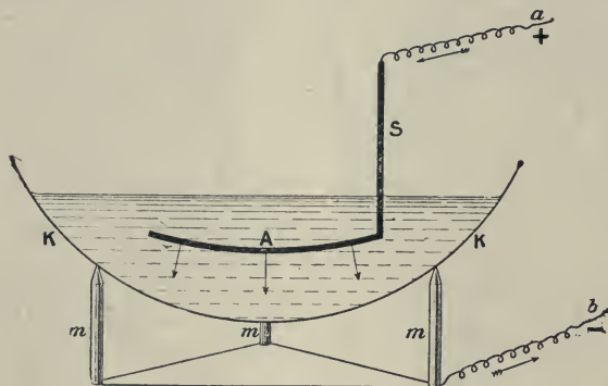
Fig. 307.—Silver Voltameter.
