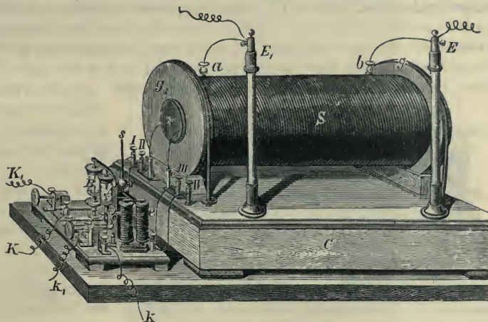
Fig. 393.—Ruhmkorff's Inductorium.
