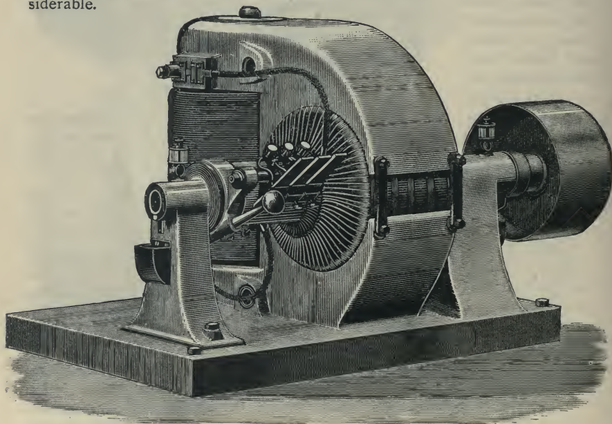
Fig. 505.—The "Leeds" Dynamo.
