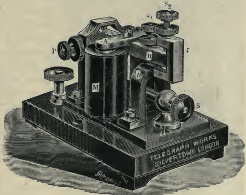
Fig. 374.—The P. O. Sounder.
