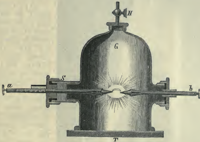
Fig. 212.—Arc Micrometer.
