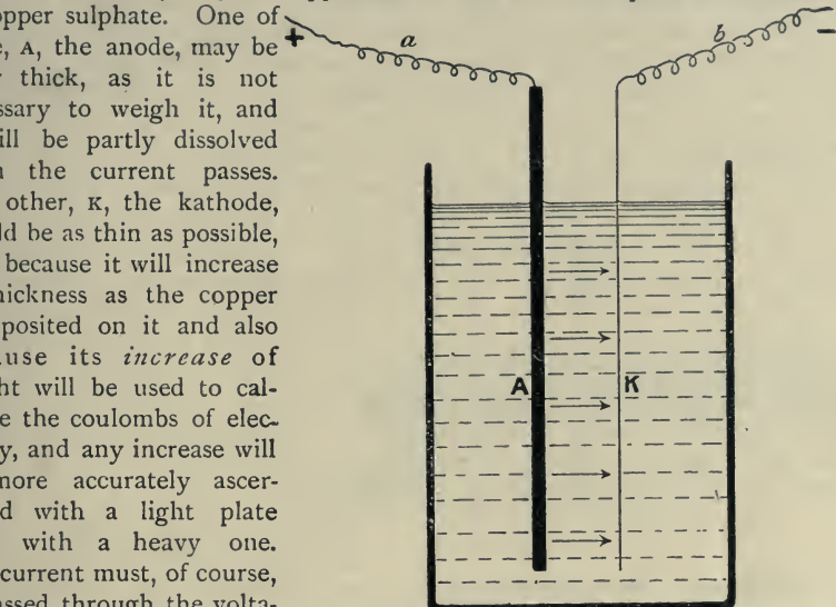
Fig. 308.—A Copper Voltameter.
