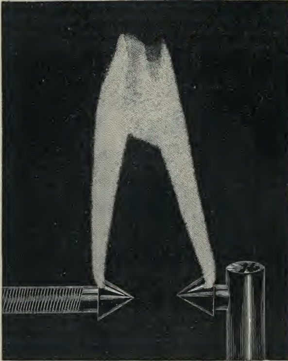
Fig. 213.—Alternate Current, 20,000 Volt Arc.
